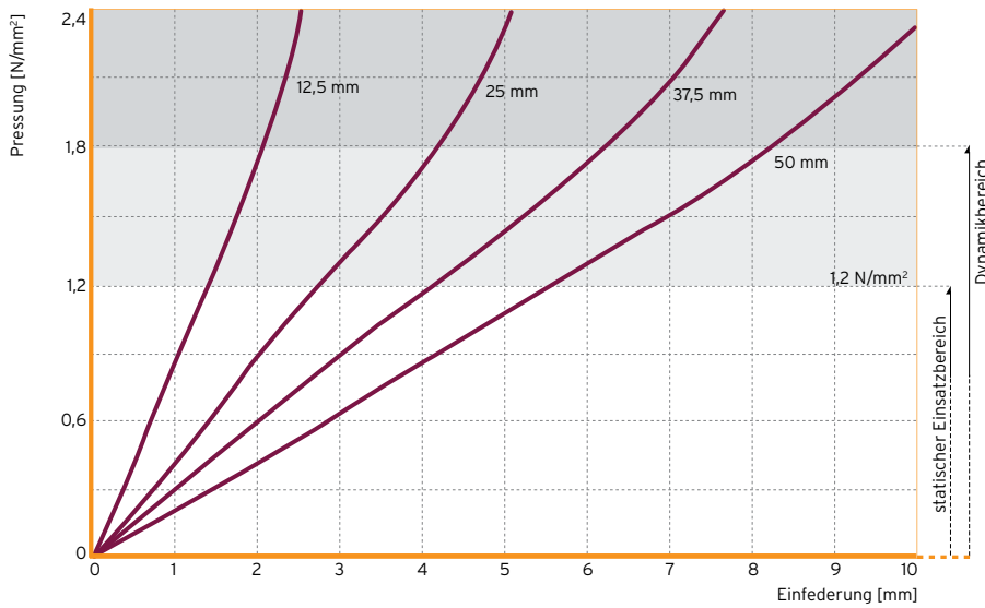
Abb. 1: Quasistatische Federkennlinie mit einer Belastungsgeschwindigkeit von 0,12 \text{ N/mm}^2/\text{s}
